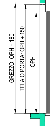
SEZIONE PORTA CON TELAIO DA 150mm
