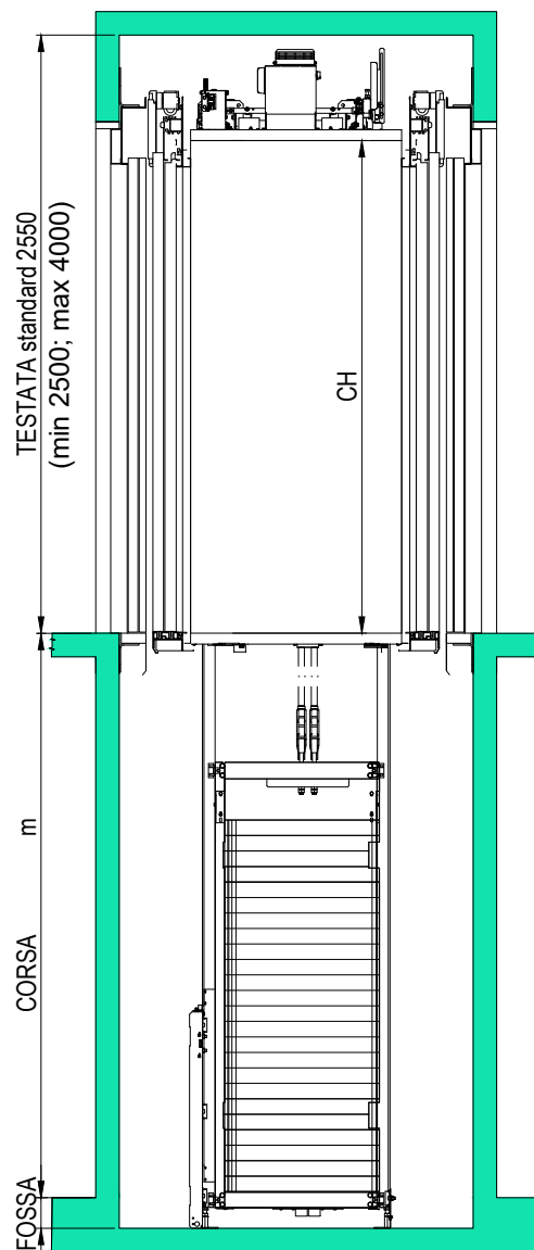
SEZIONE VANO CORSA
